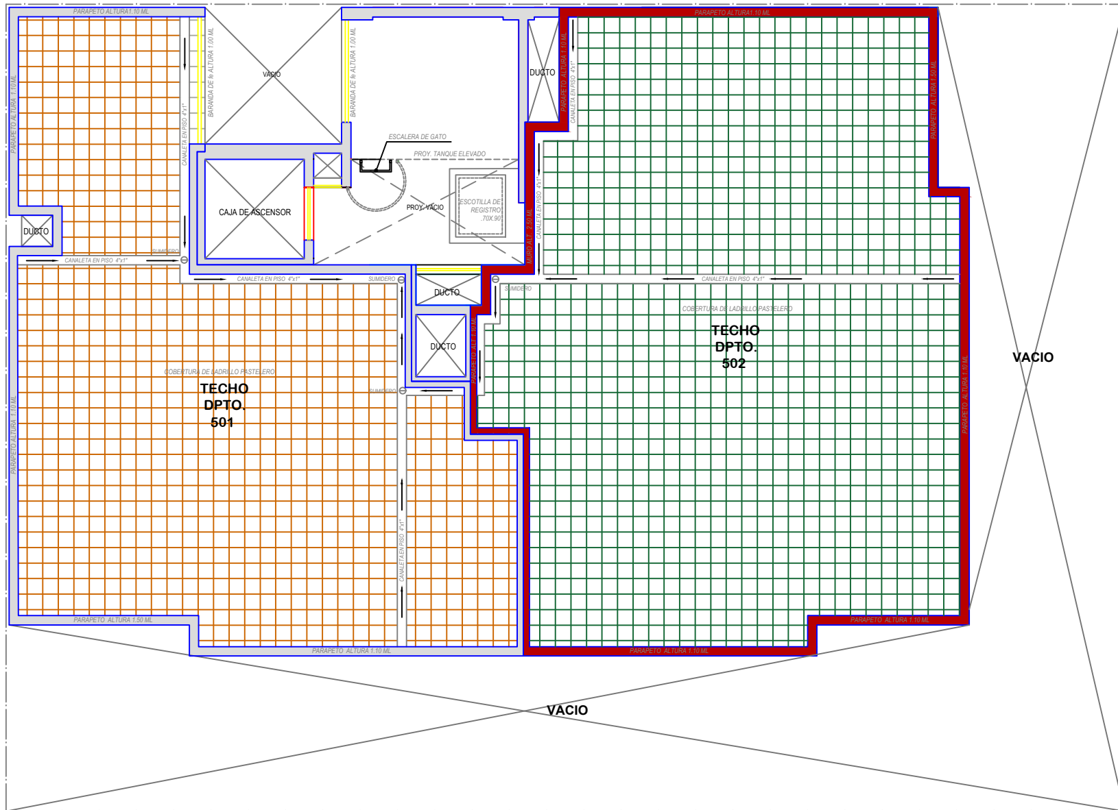
PLANTA TECHOS
